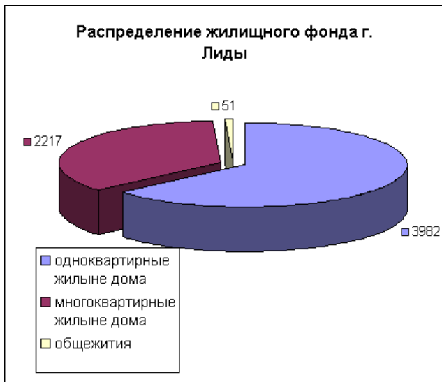
Рис. 12.1.1. Распределение жилищного фонда г. Лиды по данным на 2009 год
